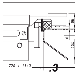
Kaavakuva 450N/5-nostimes- sa käytettävästä akselikevennin kiinnityssarjasta
